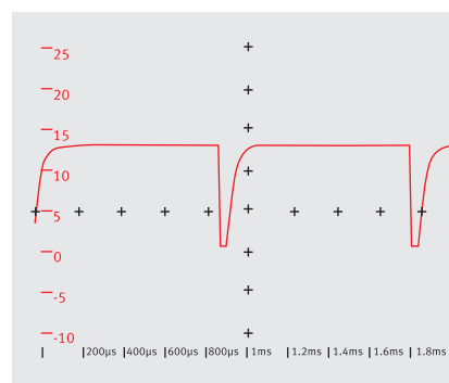
Señal en impulso de gas
