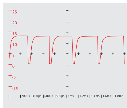
Señal en régimen de ralentí (en función de la velocidad de la marcha en ralentí)
